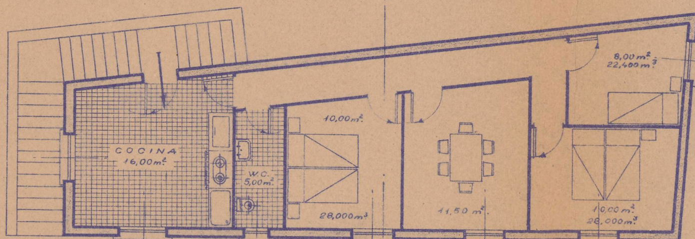
PLANTA
