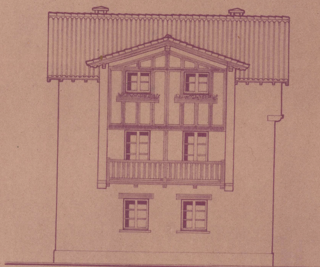
~ Fachada Sur ~
