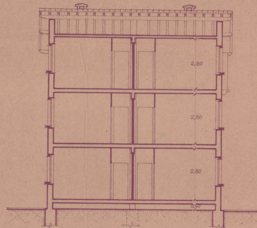
~ Sección ~
