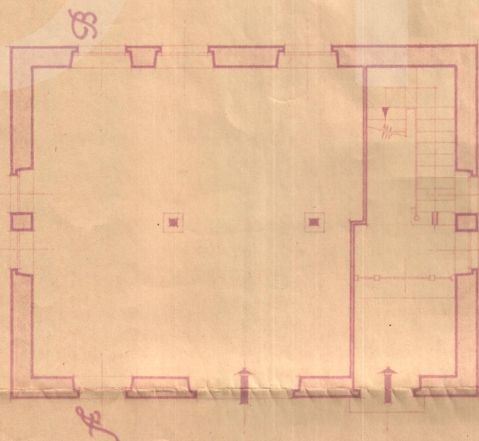
Planta baja.
