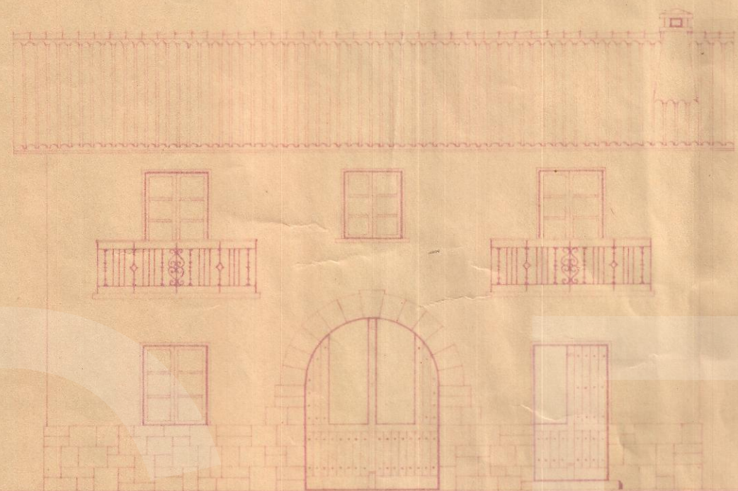
Fachada principal.
