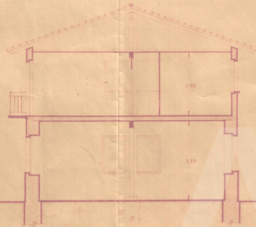
Sección A-B.
