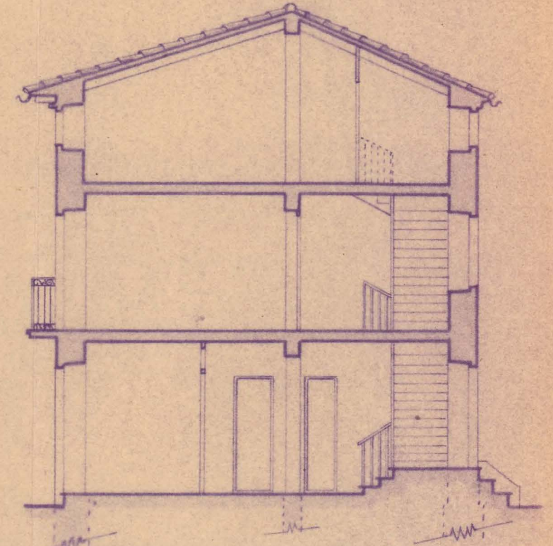
SECCION A-B.
