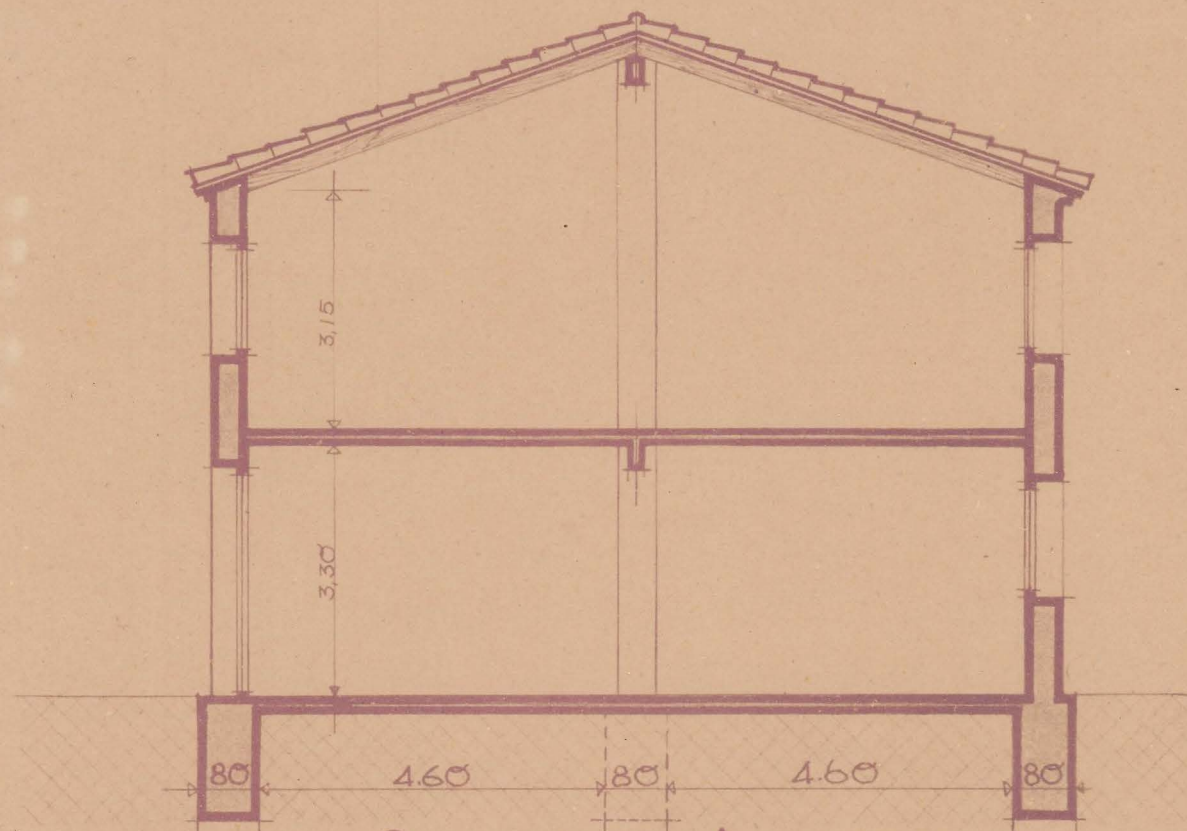
~ Sección a-b ~
