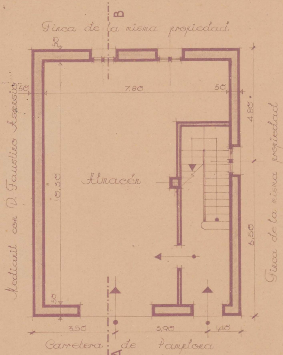
~ Planta baja ~
