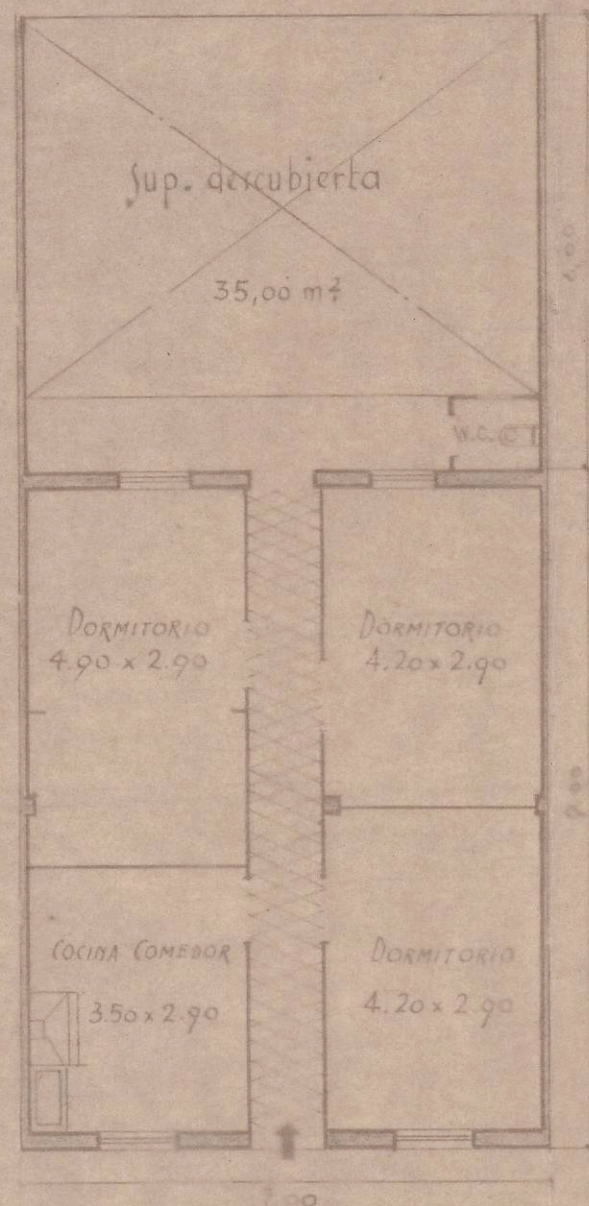
PLANTA BAJA.
