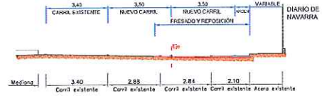
SECCION 1 - 1 E: 1/100
