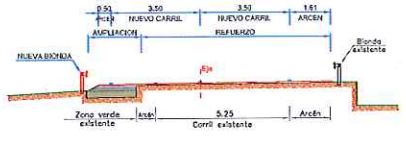
SECCION 3 - 3 E: 1/100
