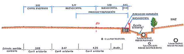
SECCION 2 - 2 E: 1/100
