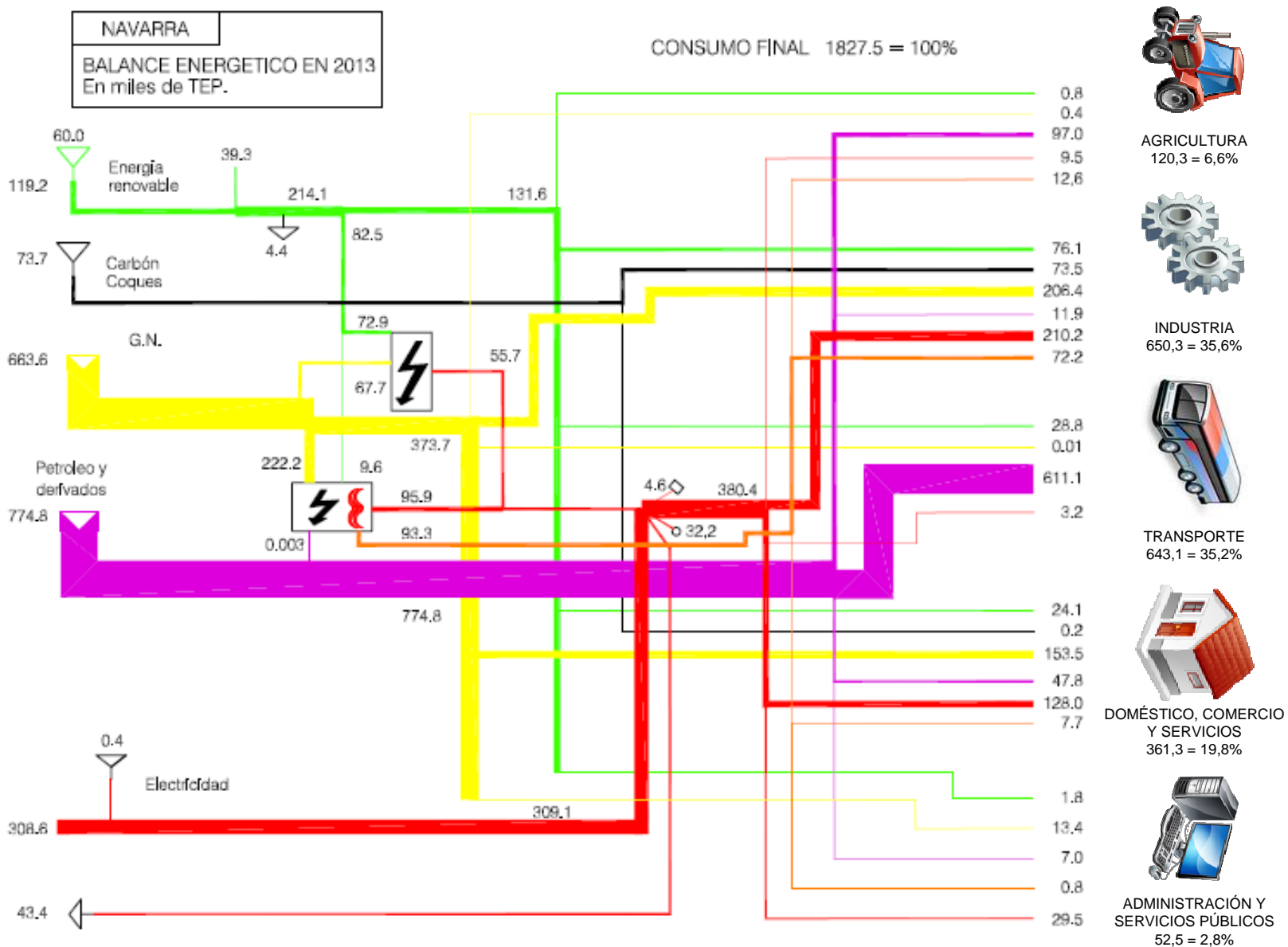
Figura 3. Representación gráfica del balance energético de Navarra 2013
