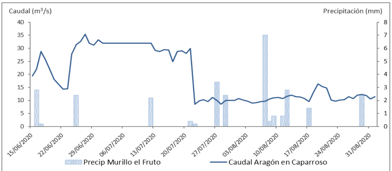
Gráfico 2. Caudales medios diarios en m³/s en la estación de aforo de Aragón en Caparroso (CHE) y precipitación acumulada diaria en l/m² en la estación meteorológica de Murillo el Fruto entre el 15-06-2020 y el 01-09-2020. Fuente de datos: Web del Agua de Navarra, MeteoNavarra y CHE. Elaboración propia. Los datos son provisionales y están sujetos a revisión.
