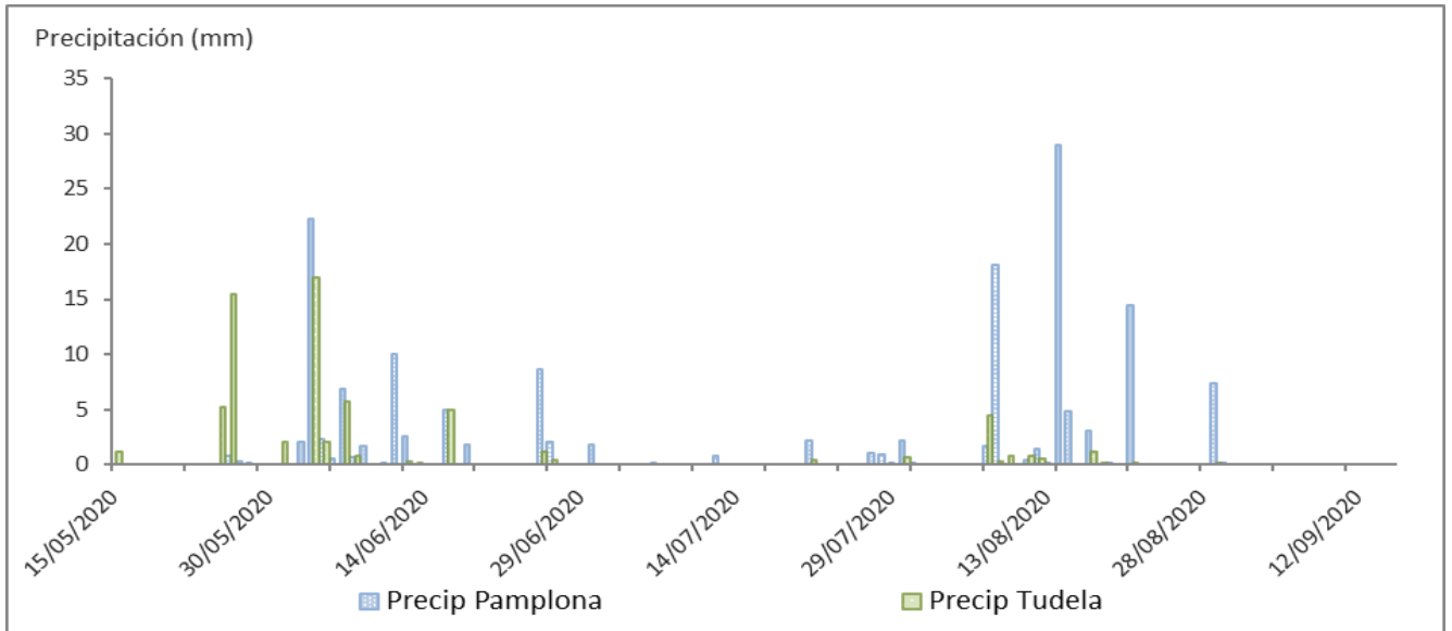
Gráfico 1. Precipitación acumulada diaria en l/m² en la estación meteorológica de Pamplona y en la de Tudela Montes del Cierzo entre el 15-05-2020 y el 15-09-2020. Fuente de datos: MeteoNavarra. Elaboración propia. Los datos son provisionales y están sujetos a revisión.
