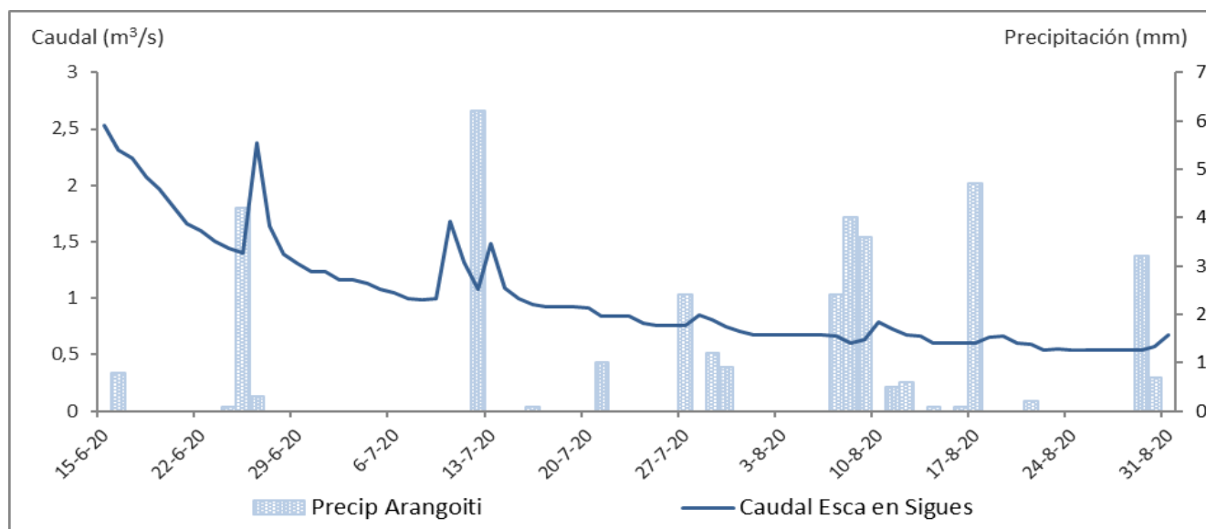
Gráfico 3. Caudales medios diarios en m 3 /s en la estación de aforo de Esca en Sigüés (CHE) y precipitación acumulada diaria en l/m 2 en la estación meteorológica de Arangoiti entre el 15-06-2020 y el 31-08-2020. Fuente de datos: Web del Agua de Navarra, MeteoNavarra y CHE. Elaboración propia. Los datos son provisionales y están sujetos a revisión.
