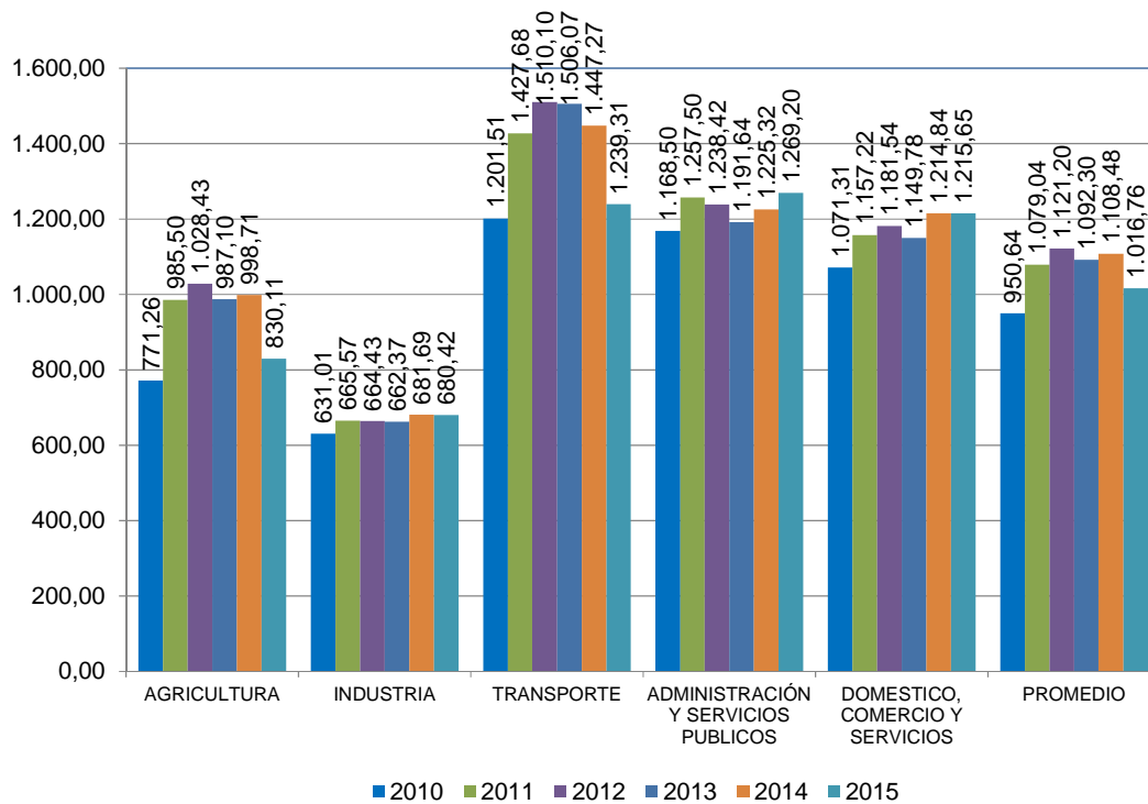
Gráfico 17. Coste de los combustibles empleados en el consumo de energía final en Navarra en 2010-2015 por sectores (euros corrientes/TEP).
