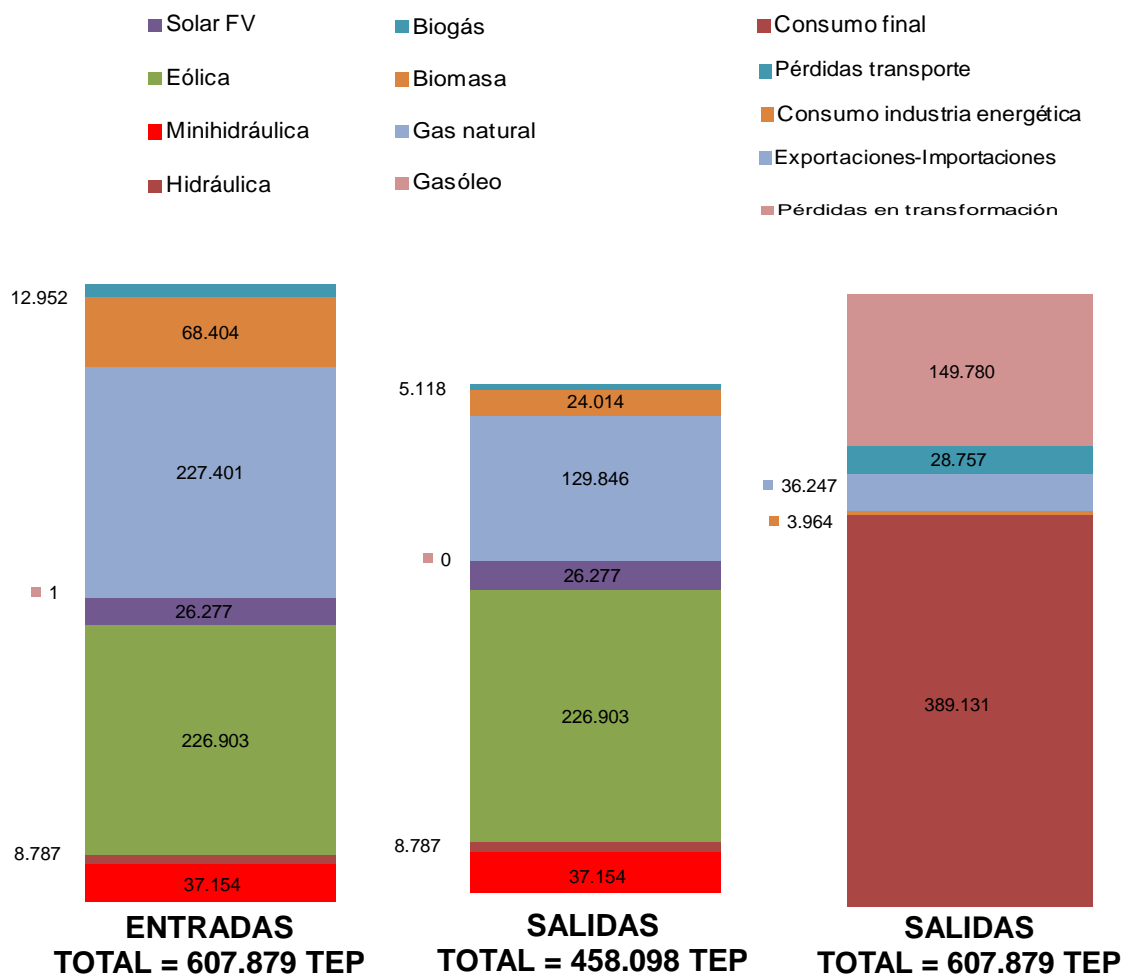
Gráfico 4. Generación eléctrica en Navarra en 2015 (TEP).
