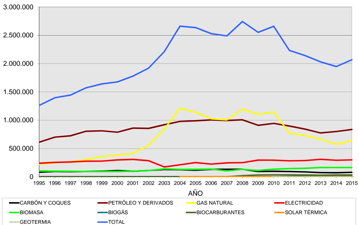
Gráfico 2. Consumo de energía primaria en Navarra 1995-2015 (TEP).
