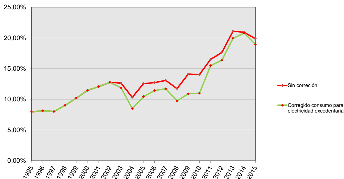
Gráfico 18. Autoabastecimiento de energía primaria (producción de energía primaria/consumo de energía primaria) (sin corrección y corregido el efecto de la electricidad excedentaria) 1995-2015
