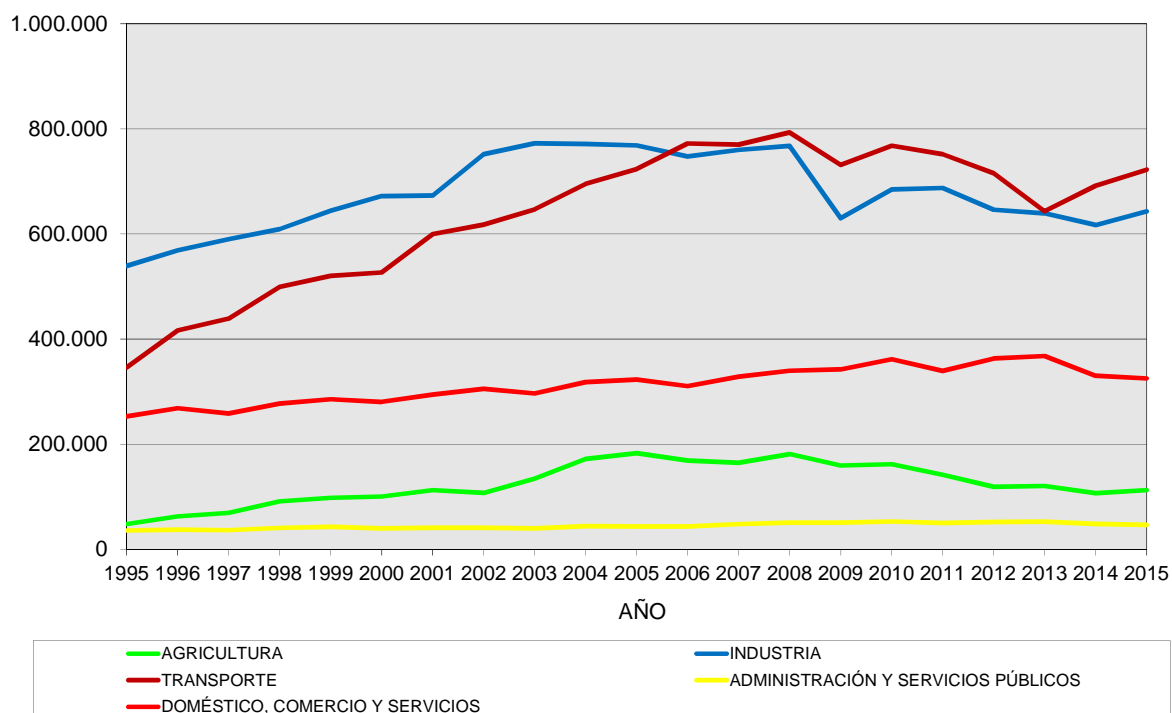
Gráfico 11. Consumo de energía final por sectores en Navarra 1995-2015 (TEP)
