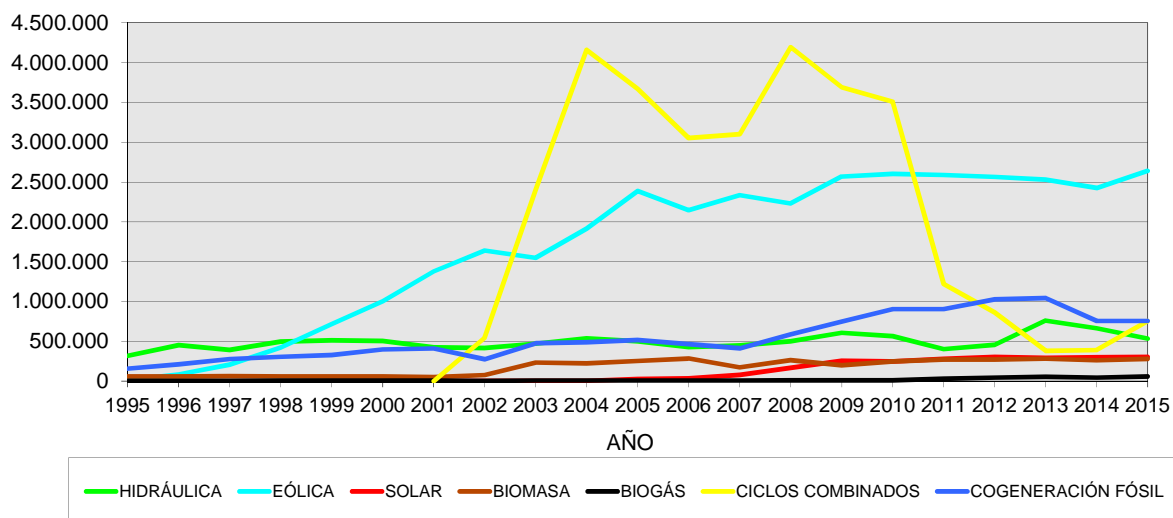
Gráfico 5. Producción eléctrica en Navarra 1995-2015 (MWh).
