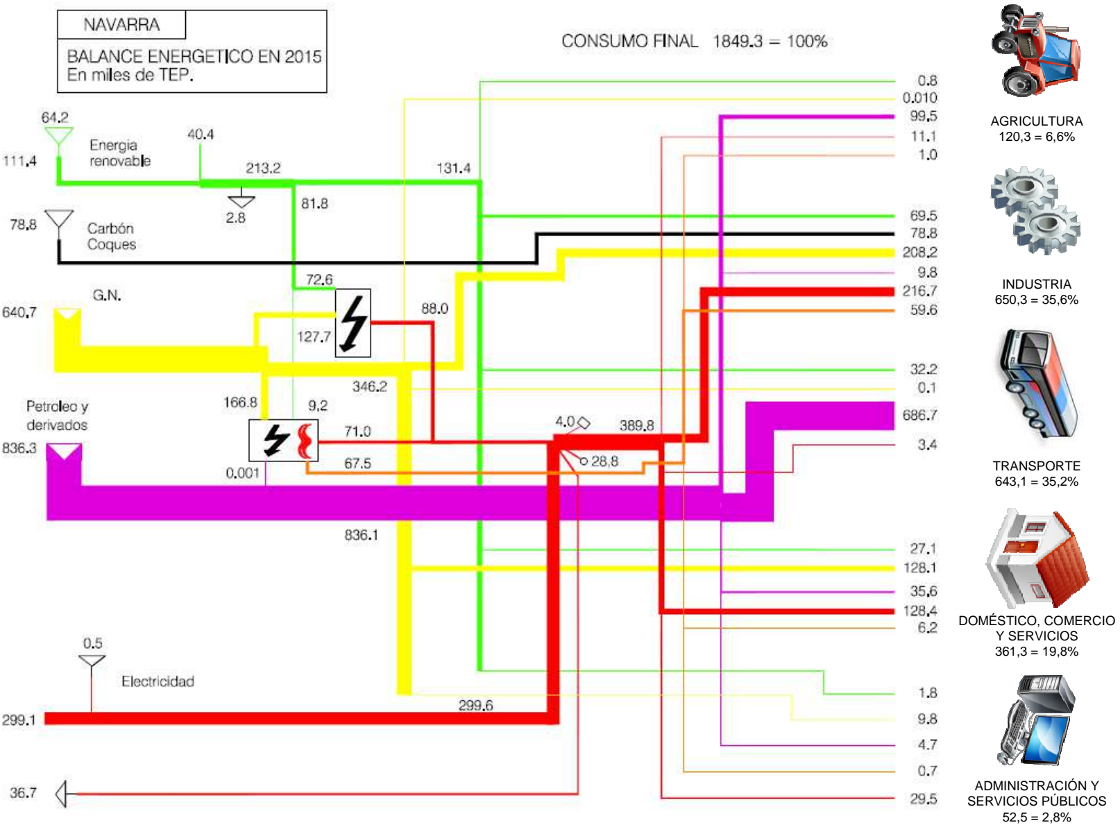
Figura 3. Representación gráfica del balance energético de Navarra 2015
