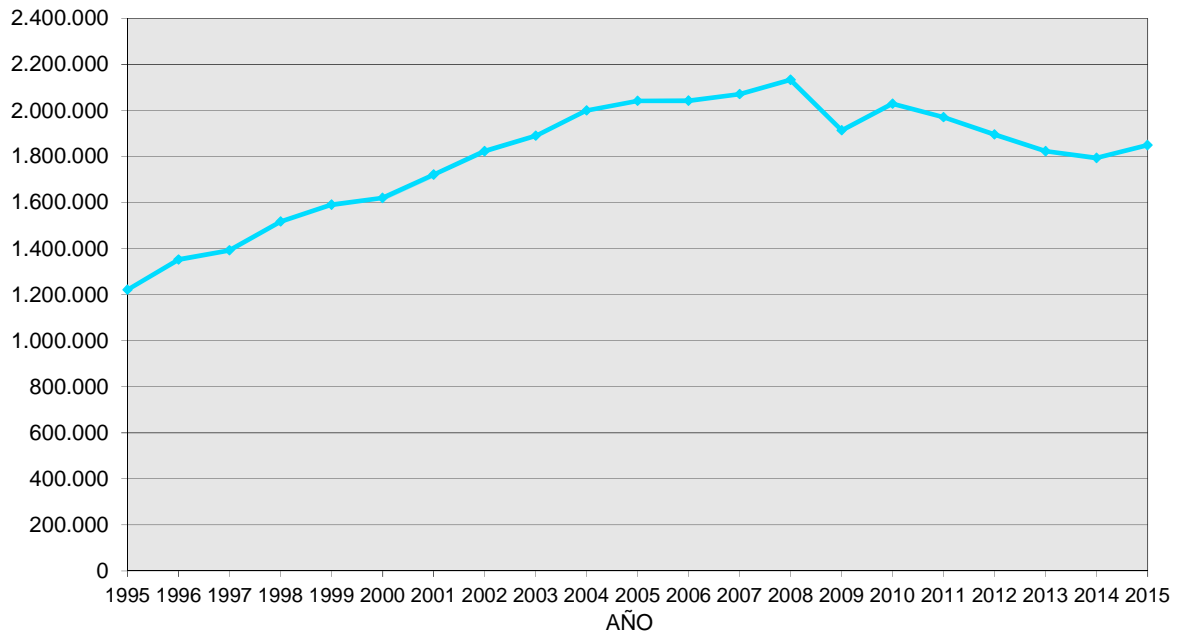
Gráfico 7. Consumo de energía final en Navarra 1995-2015 (TEP).
