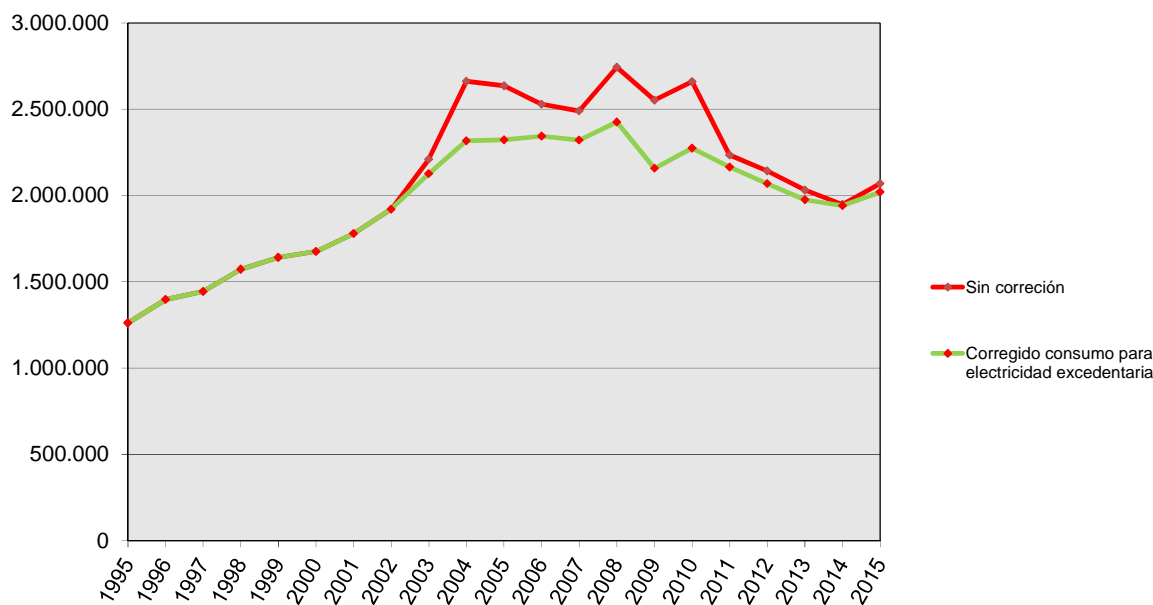
Gráfico 20. Consumo de energía primaria (sin corrección y corregido descontando el consumo para la producción de electricidad excedentaria) 1995-2015
