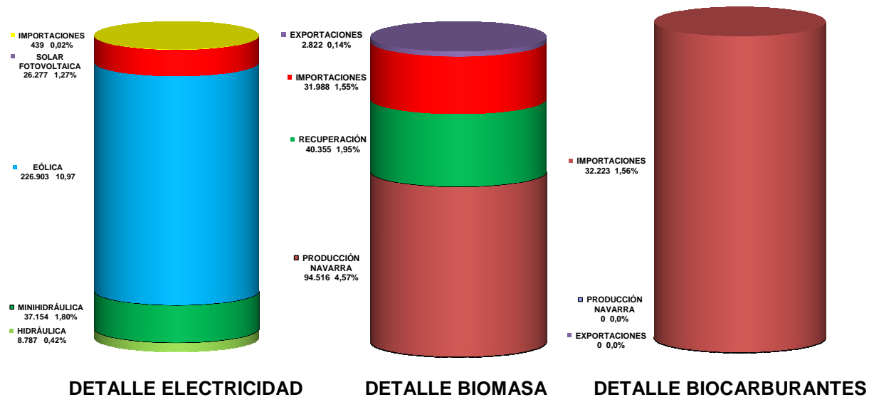
Gráfico 1. Consumo de energía primaria en Navarra en 2015 (TEP y %).
